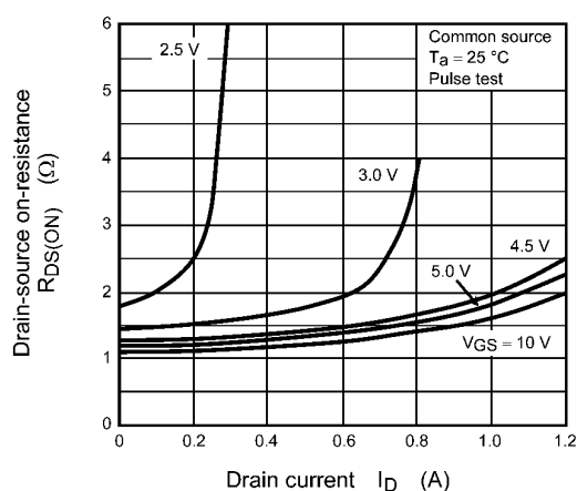
Fig. 7.3 R_{DS(ON)} - I_D
