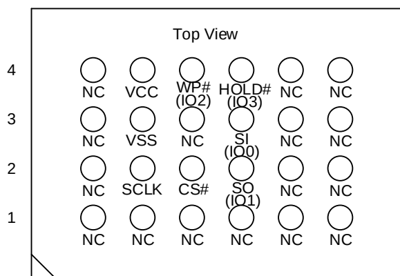
24-BALL TFBGA
