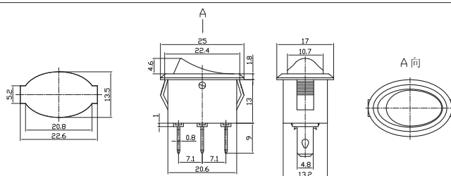
MIRS-101-10 ON-OFF 10A 125VAC;6A 250VAC SPST 3P
