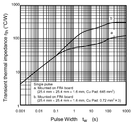
Fig. 7.13 r_{th} - t_w
