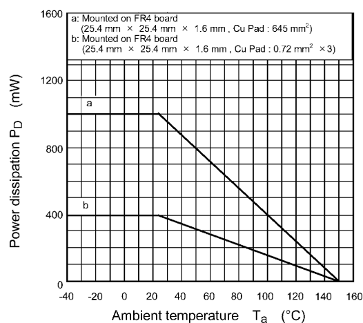
Fig. 7.14 P_D - T_a
