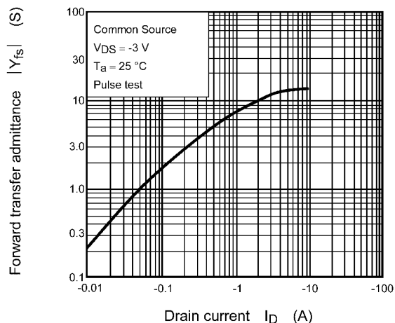
Fig. 7.8 |Y_{fs}| - I_D
