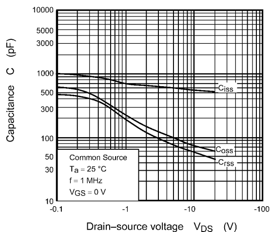
Fig. 7.10 C - V_{DS}
