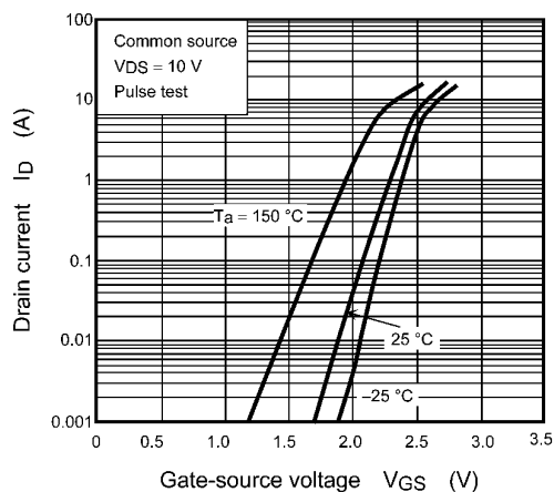
Fig. 8.2 I_D - V_{GS}
