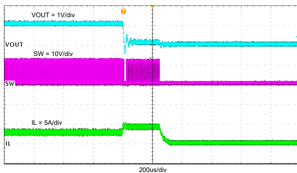
图 7-16. TPS562243 正常运行至输出硬短路
