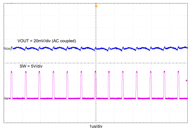
图 7-4. TPS562243 输出电压纹波 (2A 负载)
