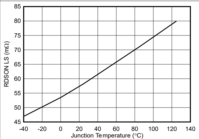
图 5-6. 高侧 Rdson
