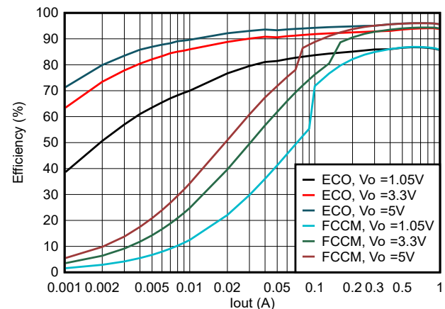
TPS56124x 在 V_{in} = 12V 时的效率
