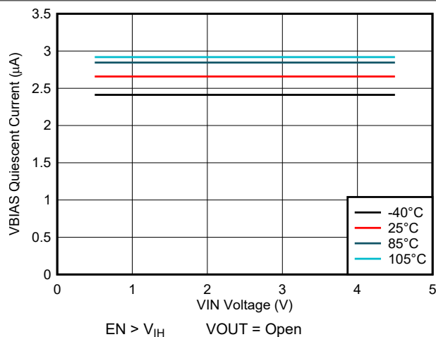
图 5-3. VBIAS Quiescent Current vs VIN Voltage
