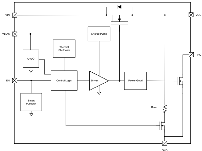
TPS22999 方框图
