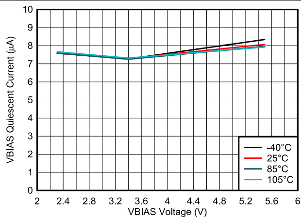
图 5-2. VBIAS Quiescent Current vs VBIAS Voltage
