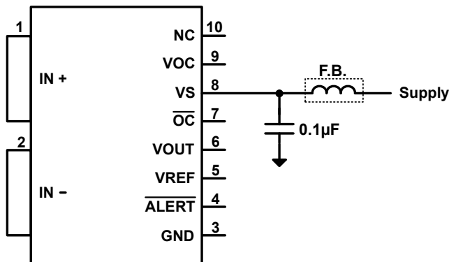
图 9-4. 电源噪声滤波
