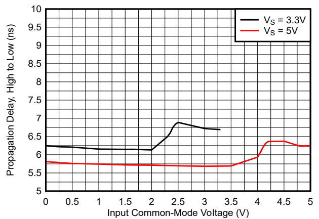
图 5-18. 传播延迟 (高电平到低电平) 与共模电压间的关系
