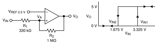
图 7-5. 采用非反相配置、具有迟滞功能的 TLV3231
