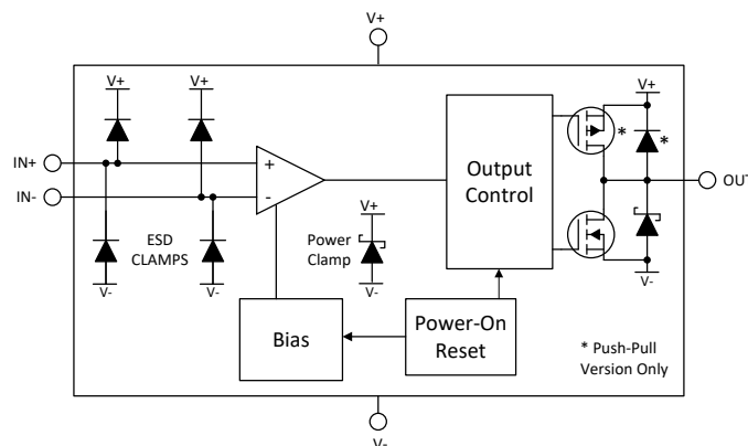
TLV18xx-Q1 方框图
