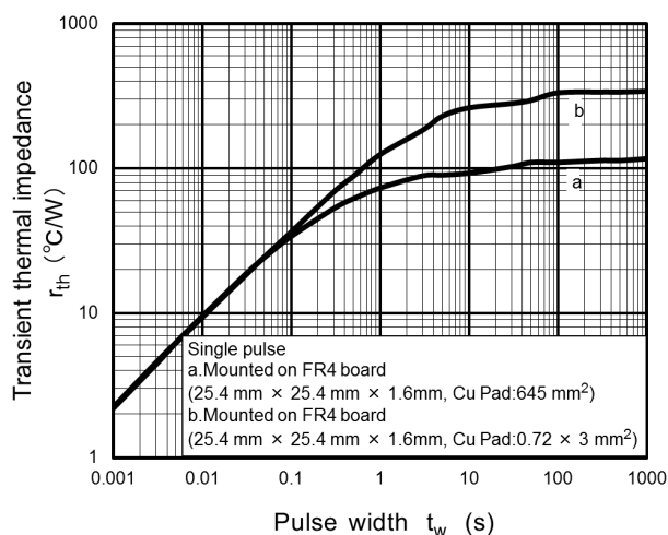
Fig. 7.11 r_{th} - t_w
