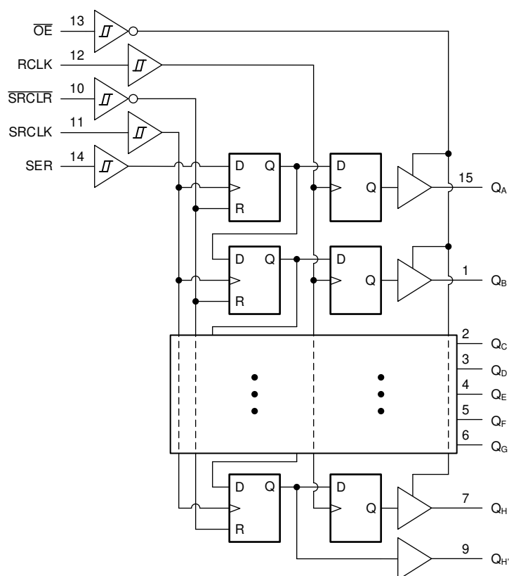
图 7-1. SN74LV8T595 的逻辑图 (正逻辑)
