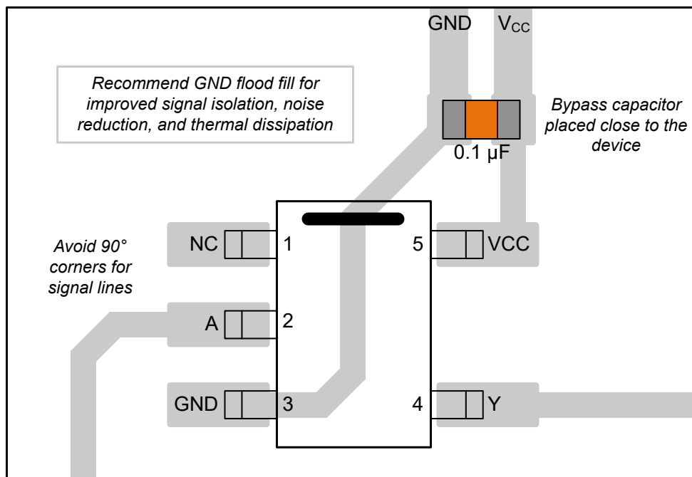
图 9-3. SN74AHC1G14-Q1 的示例布局
