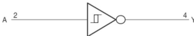
简化逻辑图 (正逻辑)
