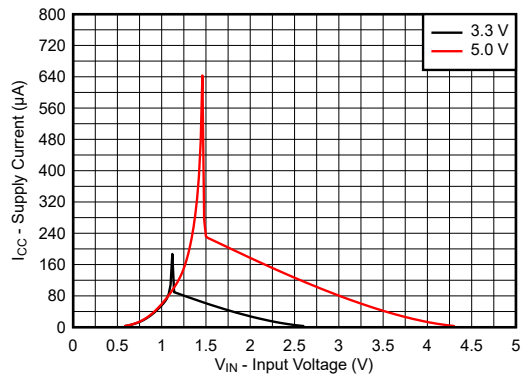
图 6-1. 3.3V 和 5.0V 输入电压电源上的电源电流
