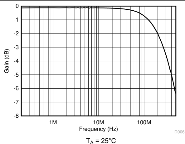
图 5-4. 频率响应
