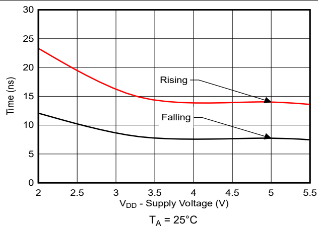
图 5-2. T_{\text{transition}} 与电源电压之间的关系
