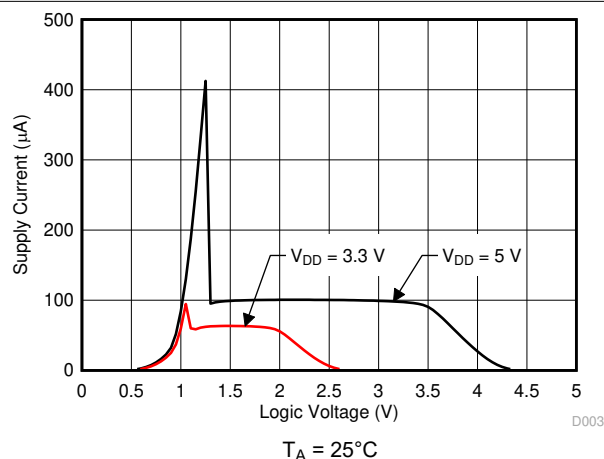
图 5-1. 电源电流与逻辑电压间的关系
