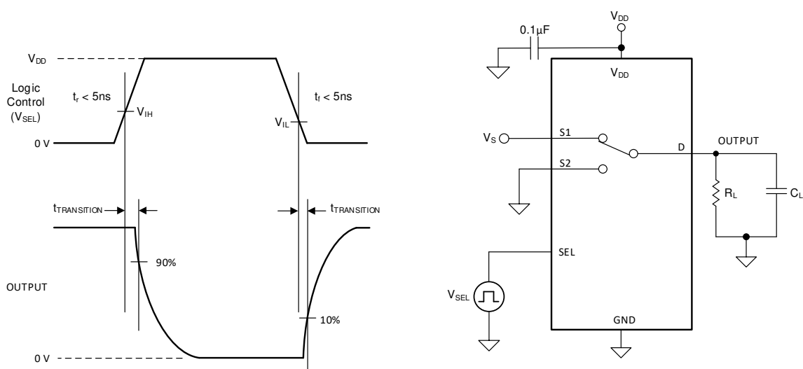
图 6-4. 转换时间测量设置
