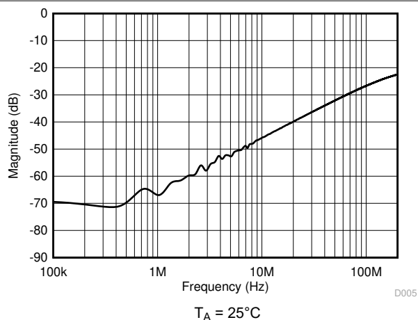
图 5-3. 串扰和关断隔离与频率之间的关系
