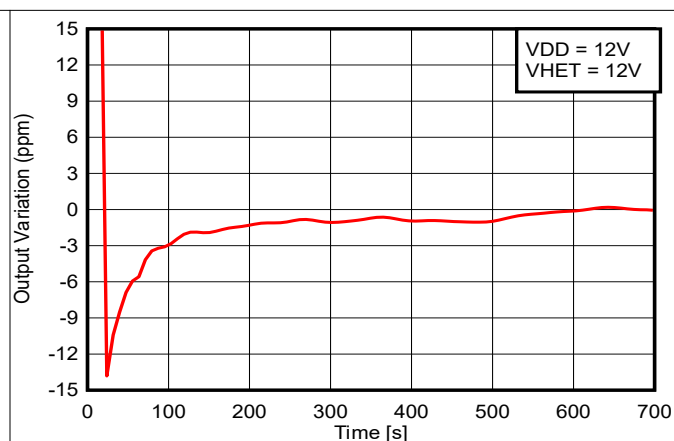
图 6-14. 启动行为
