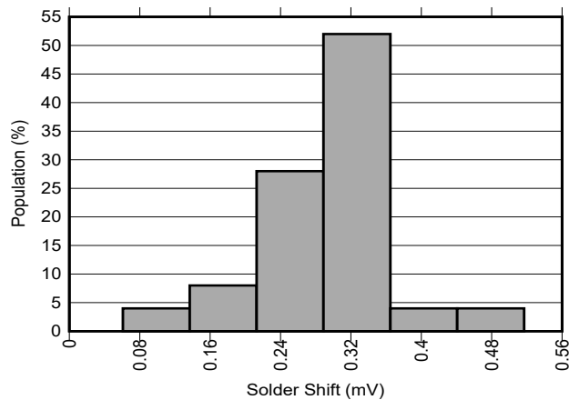
图 6-11. 焊接移位分布
