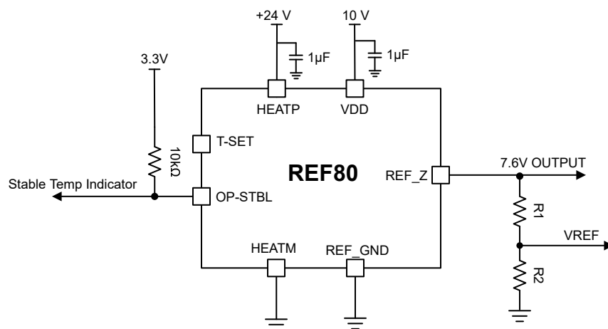
图 9-3. 精密电阻分压器连接
