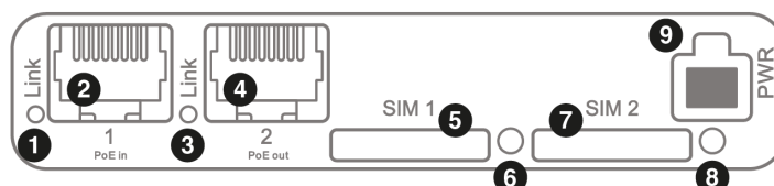
Рис. 2. Вид спереди R11-A.W
