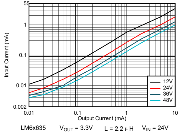
图 8-44. 输入电源电流 - 自动模式
