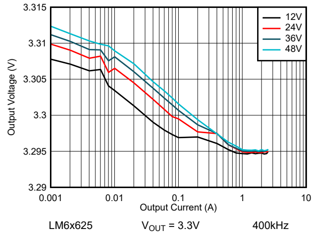
图 8-20. LM6x625 线路和负载调节 - 自动模式
