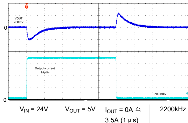
图 8-63. 负载瞬态 - LM6x635 - FPWM
