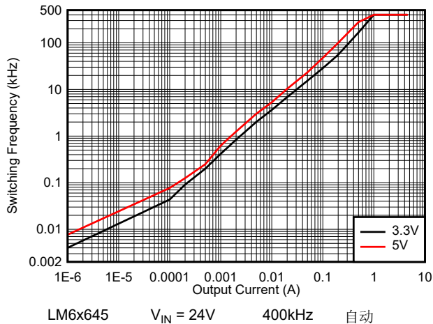
图 8-33. LM6x645 开关频率与负载电流间的关系
