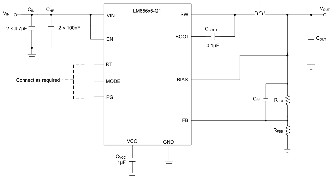
图 8-1. LM656x5-Q1 可调输出电压模式下的示例应用电路
