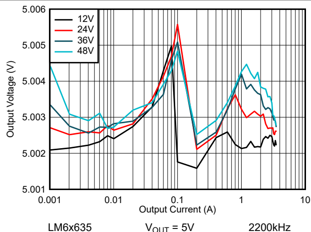
图 8-25. LM6x635 线路和负载调节 - 自动模式
