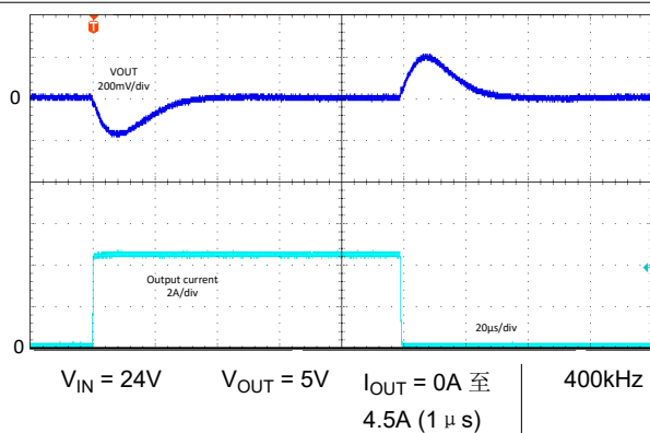
图 8-65. 负载瞬态 - LM6x645 - FPWM
