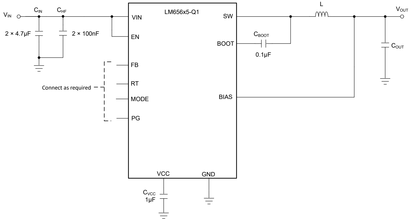
图 8-2. LM656x5-Q1 固定输出电压模式下的示例应用电路
