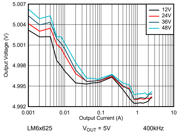
图 8-19. LM6x625 线路和负载调节 - 自动模式
