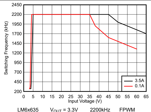
图 8-36. LM6x635 开关频率与输入电压间的关系
