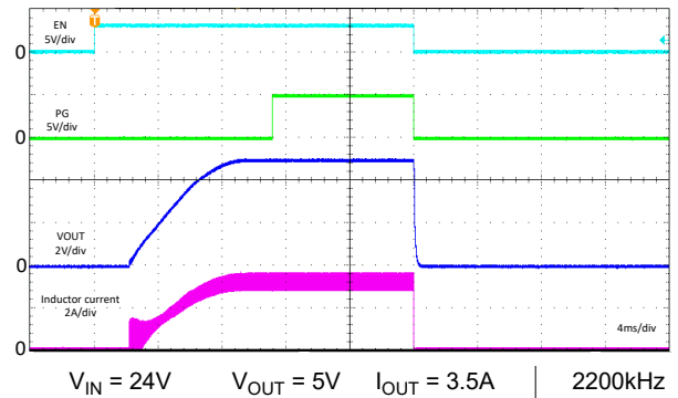
图 8-68. 启动/关断 - FPWM
