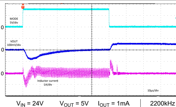
图 8-71. 模式变化瞬态
