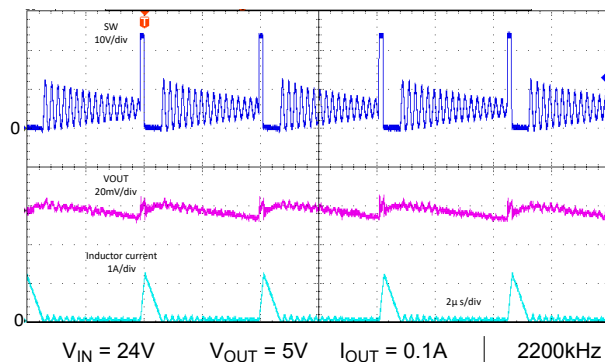
图 8-62. 典型开关波形 - LM6x625 - 自动
