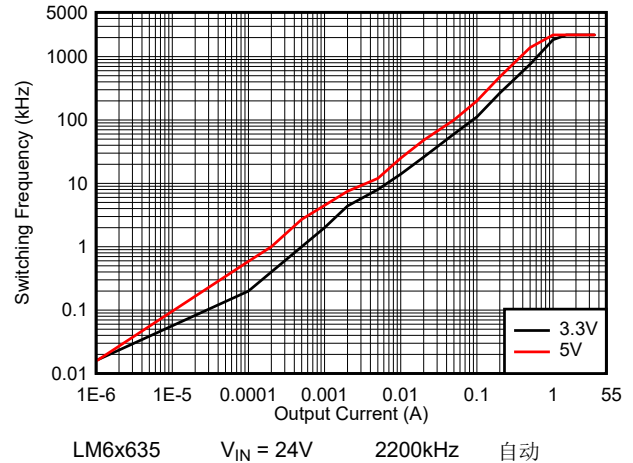
图 8-32. LM6x635 开关频率与负载电流间的关系
