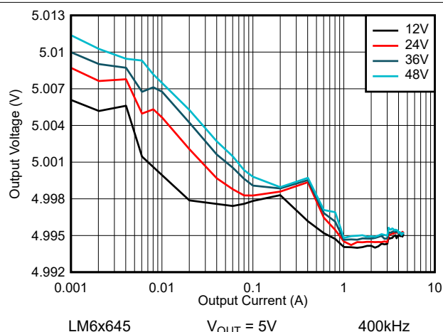
图 8-27. LM6x645 线路和负载调节 - 自动模式
