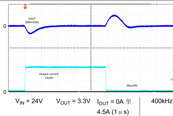
图 8-66. 负载瞬态 - LM6x645 - FPWM
