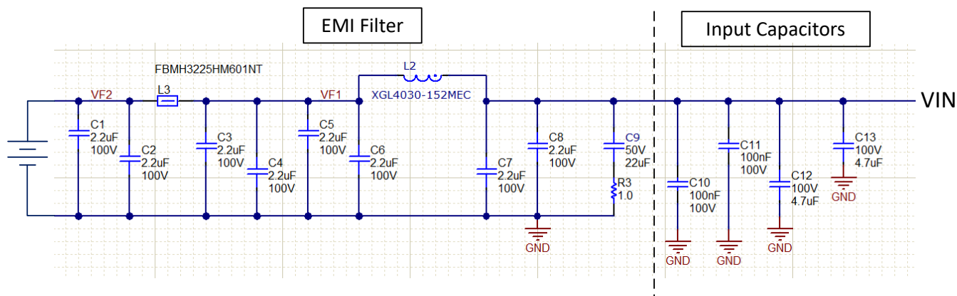
图 8-75. 适用于 2200kHz 的 EMI 输入滤波器
