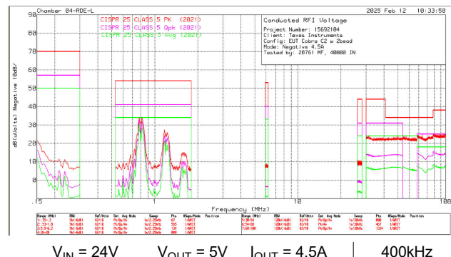
图 8-58. LM6x645 传导 EMI - 负向线路
