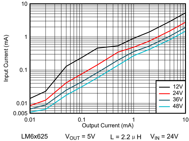
图 8-43. 输入电源电流 - 自动模式
