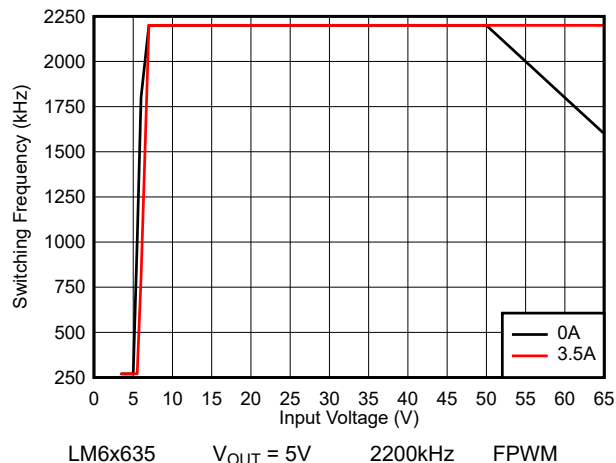
图 8-37. LM6x635 开关频率与输入电压间的关系
