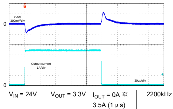
图 8-64. 负载瞬态 - LM6x635 - FPWM
