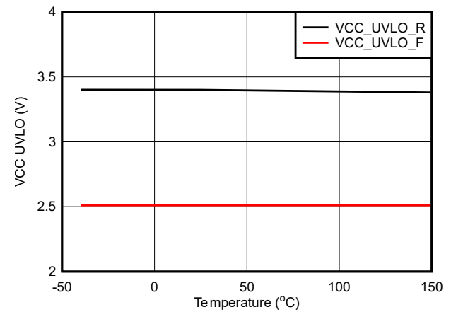
图 6-4. VCC UVLO
