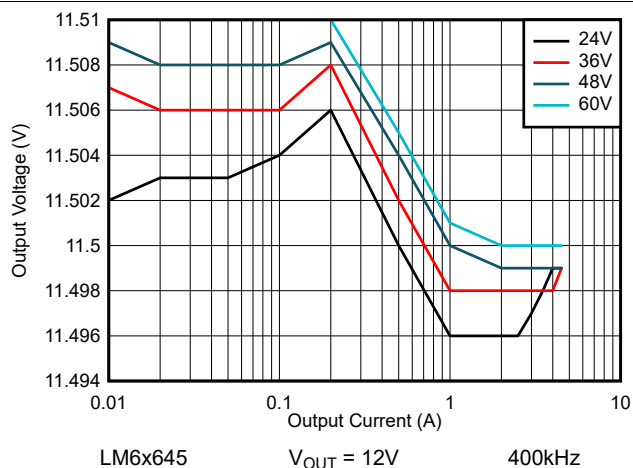
图 8-52. LM6x645 线路和负载调节 - V_{OUT} = 12V - 自动模式
