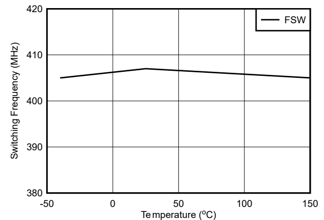
图 6-6. f_{SW} 400kHz
