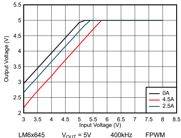
图 8-38. LM6x645 压降特性
