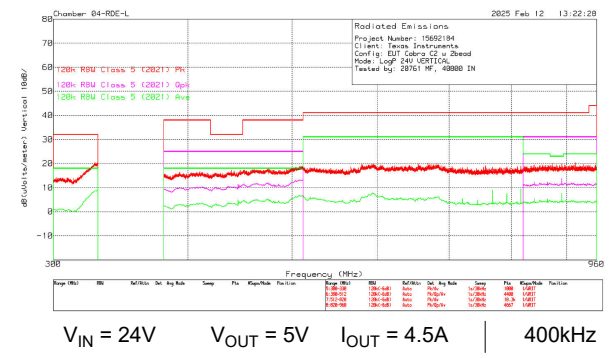
图 8-60. LM6x645 辐射 EMI - 对数周期 - 垂直
