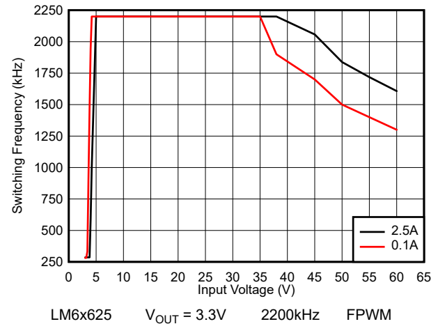
图 8-34. LM6x625 开关频率与输入电压间的关系
