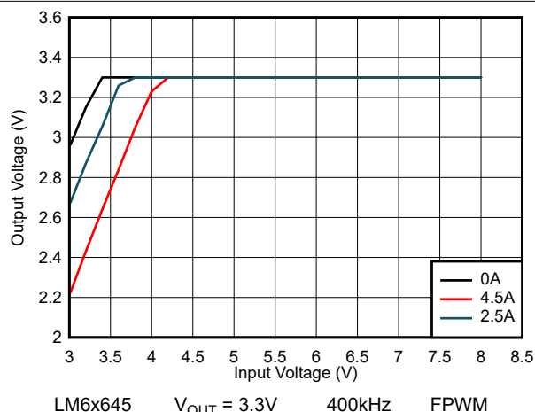
图 8-39. LM6x645 压降特性
