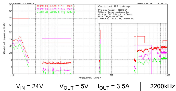
图 8-54. LM6x635 传导 EMI - 负向线路
