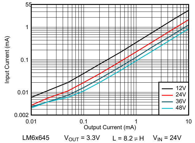
图 8-46. 输入电源电流 - 自动模式
