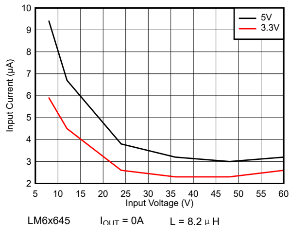
图 8-50. 空载输入电源电流 - 自动模式
