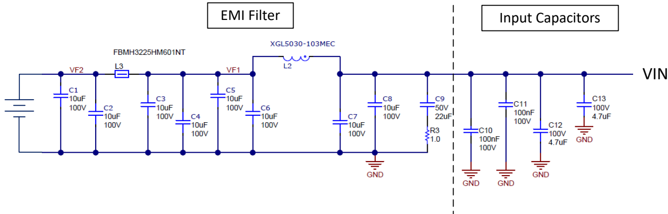
图 8-76. 适用于 400kHz 的 EMI 输入滤波器
