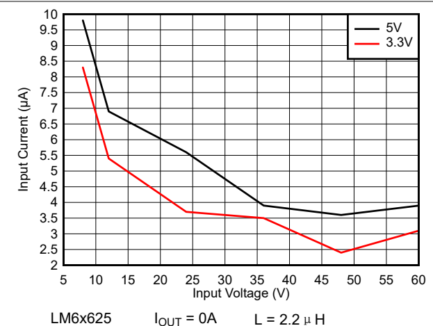
图 8-48. 空载输入电源电流 - 自动模式
