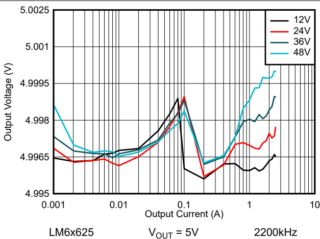
图 8-21. LM6x625 线路和负载调节 - 自动模式
