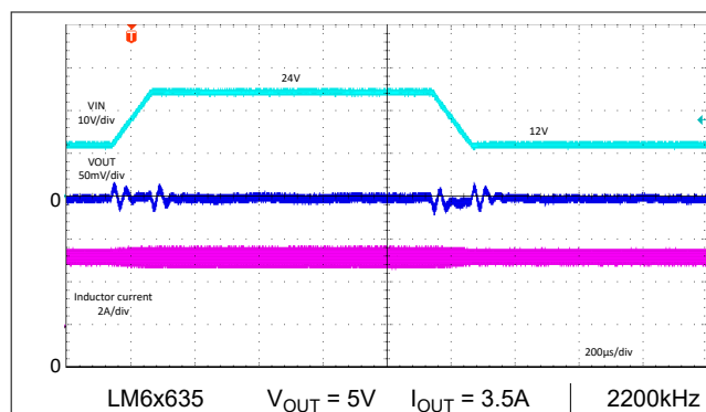
图 8-73. 线路瞬态 - 自动
