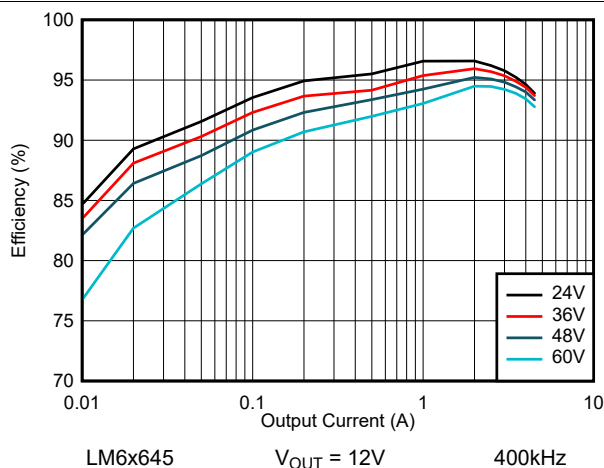
图 8-51. LM6x645 效率 - V_{OUT} = 12V - 自动模式
