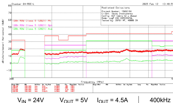
图 8-59. LM6x645 辐射 EMI - 对数周期 - 水平
