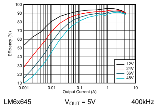
图 3-1. LM6x645 效率 - 自动模式
