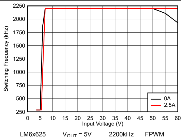
图 8-35. LM6x625 开关频率与输入电压间的关系
