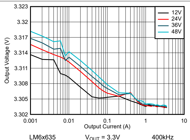
图 8-24. LM6x635 线路和负载调节 - 自动模式
