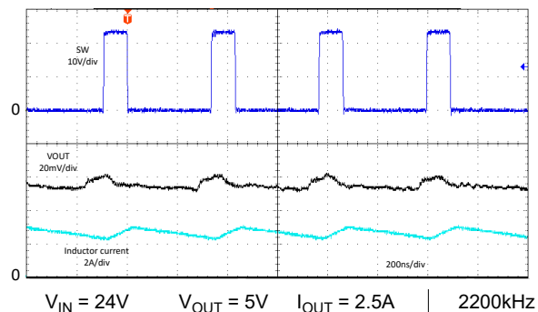
图 8-61. 典型开关波形 - LM6x625 - FPWM
