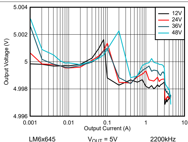
图 8-29. LM6x645 线路和负载调节 - 自动模式
