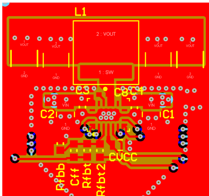
图 8-78. 布局示例
