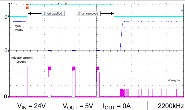
图 8-69. 输出短路电路和恢复 - 自动
