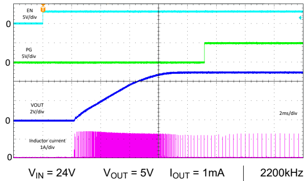
图 8-67. 启动 - 自动
