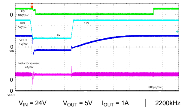
图 8-72. 压降瞬态和恢复
