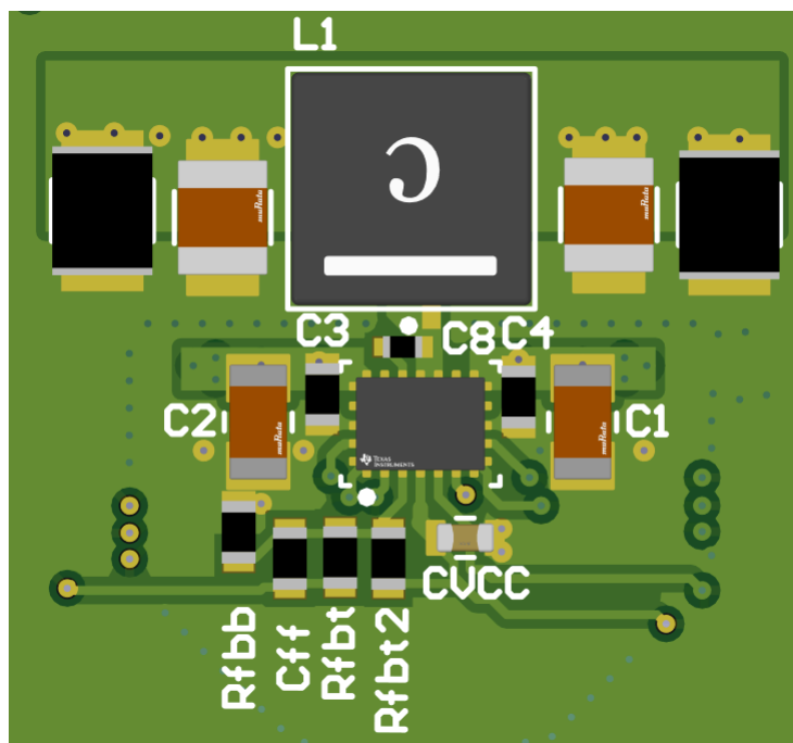
图 8-79. PCB 图像
