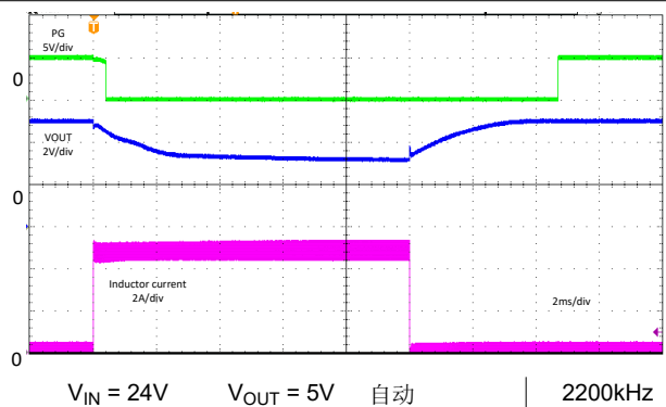
图 8-70. 电流限值瞬态
