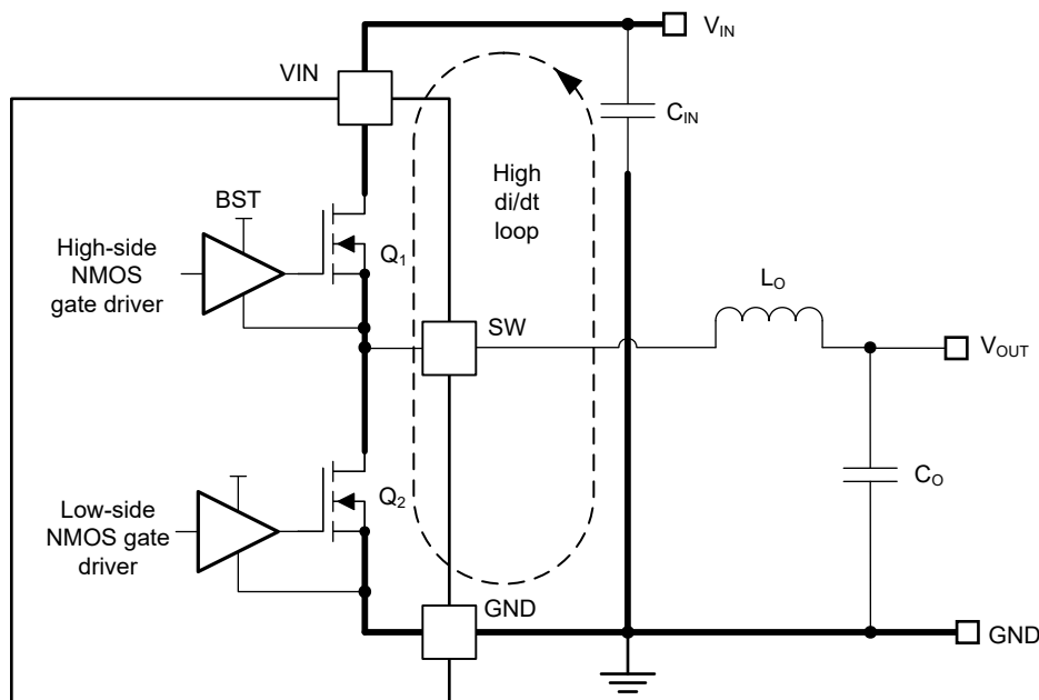
图 8-77. 具有快速边沿的电流环路
