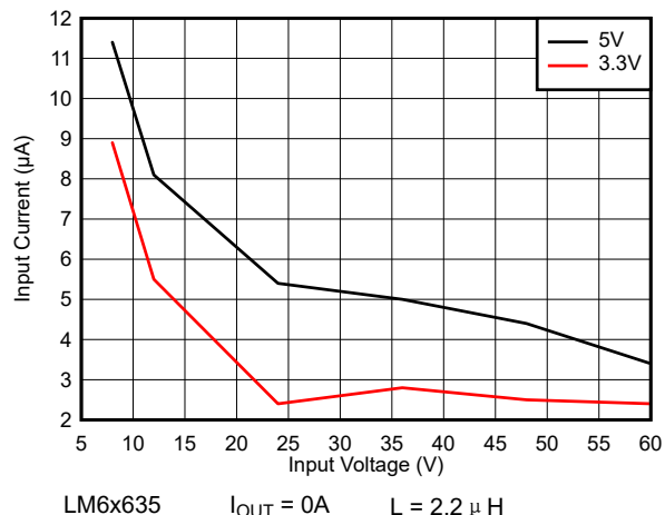
图 8-49. 空载输入电源电流 - 自动模式
