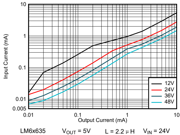
图 8-45. 输入电源电流 - 自动模式
