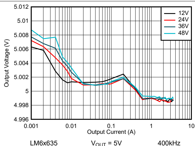
图 8-23. LM6x635 线路和负载调节 - 自动模式
