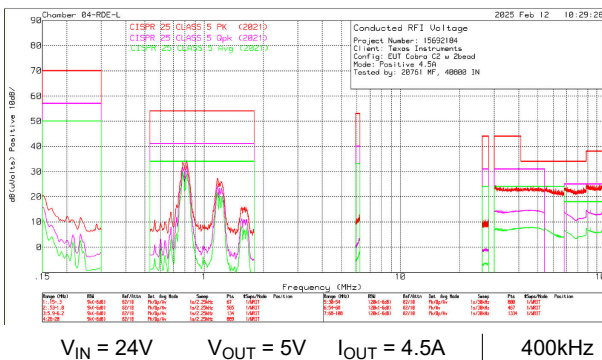
图 8-57. LM6x645 传导 EMI - 正向线路
