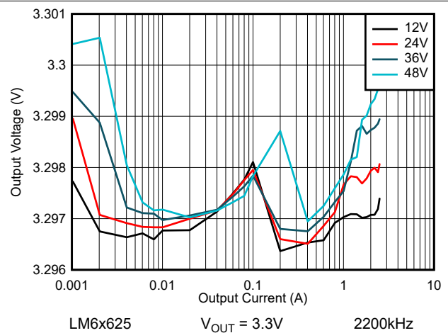
图 8-22. LM6x625 线路和负载调节 - 自动模式
