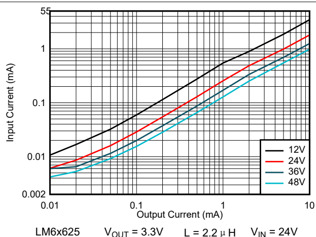
图 8-42. 输入电源电流 - 自动模式
