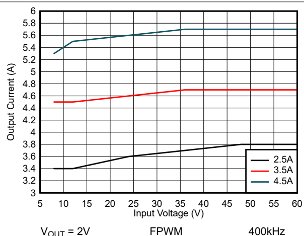
图 8-41. 最大输出电流
