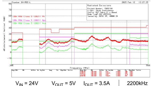
图 8-56. LM6x635 辐射 EMI - 对数周期 - 垂直
