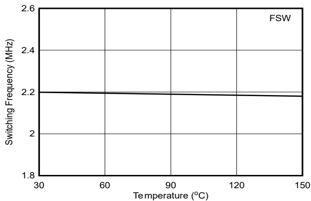
图 6-5. f_{SW} 2.2MHz
