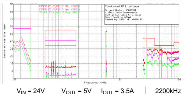
图 8-53. LM6x635 传导 EMI - 正向线路
