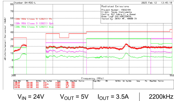
图 8-55. LM6x635 辐射 EMI - 对数周期 - 水平
