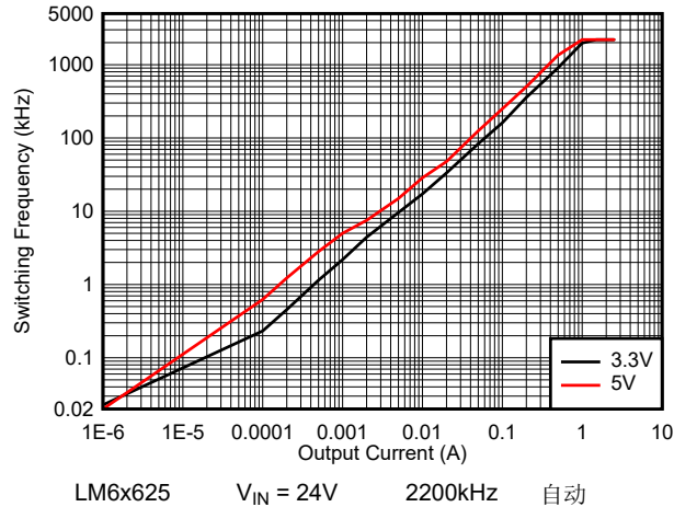
图 8-31. LM6x625 开关频率与负载电流间的关系
