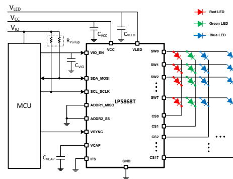
简化原理图
