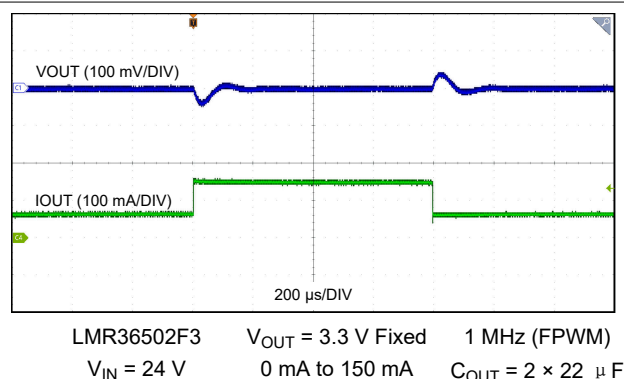
图 9-8. Load Transient
