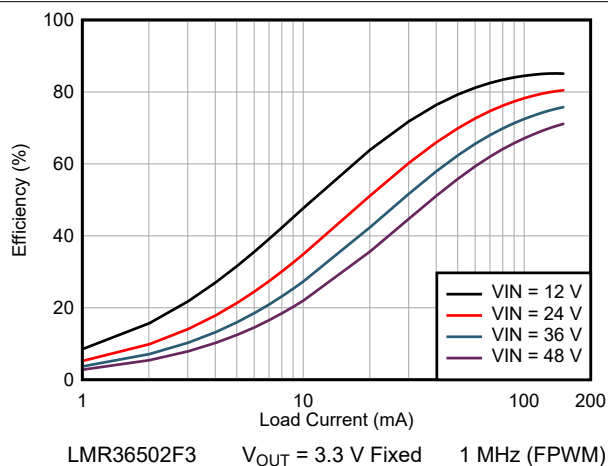
图 9-3. Efficiency
