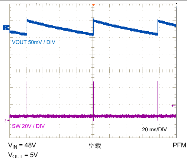
图 7-16. PFM 开关
