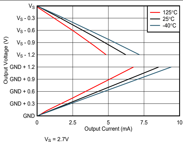
图 6-22. 输出电压与输出电流间的关系
