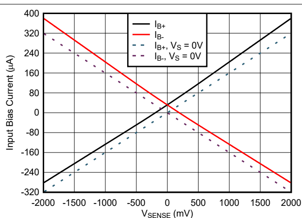
图 6-18. INA296x-Q1 输入偏置电流与 V_{\text{SENSE}} 间的关系
