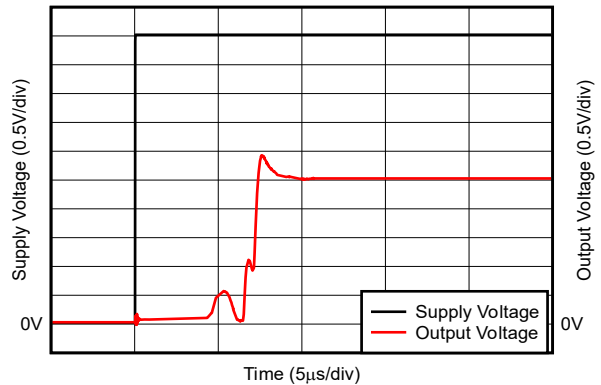
图 6-34. 小阶跃响应
