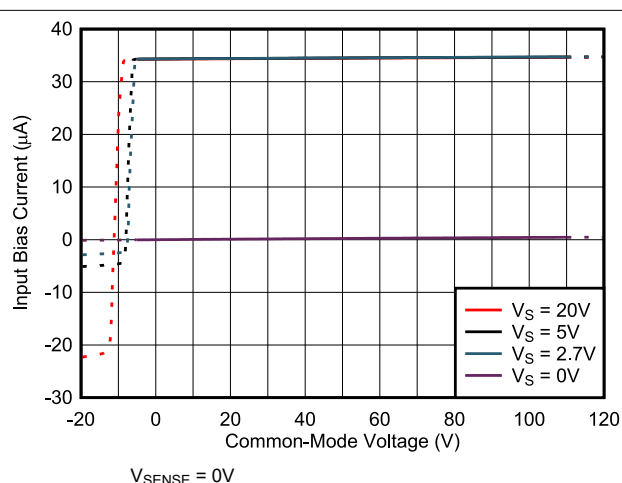
图 6-16. 输入偏置电流与共模电压间的关系
