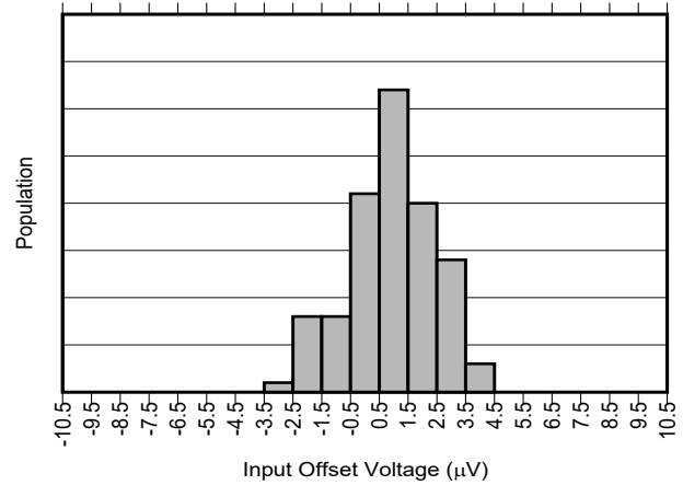
图 6-2. INA296A2-Q1 输入失调电压产生分布图
