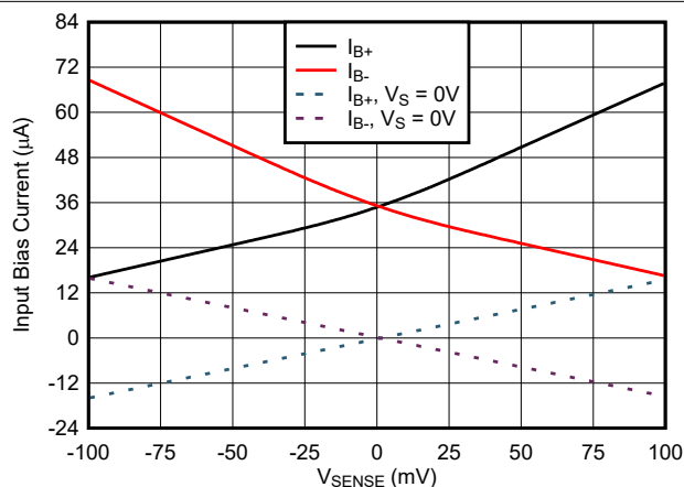
图 6-21. INA296 x5-Q1 输入偏置电流与 V_{\text{SENSE}} 间的关系
