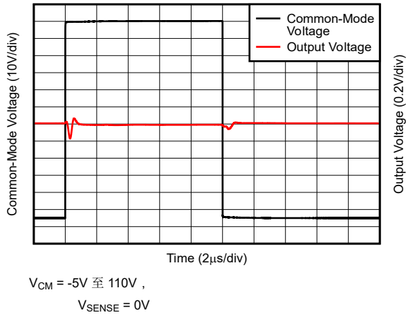
图 6-33. 共模电压快速瞬态脉冲
