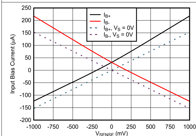
图 6-19. INA296x1-Q1 输入偏置电流与 V_{\text{SENSE}} 间的关系
