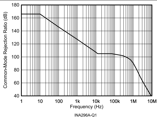
图 6-8. 共模抑制比与频率间的关系
