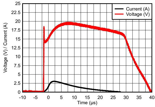
图 5-7. 8/20 \mu s 浪涌响应
